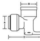
垂耳式弯头尺寸
