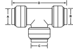
三通尺寸
