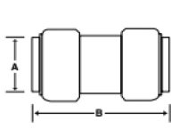
直式耦合头尺寸
